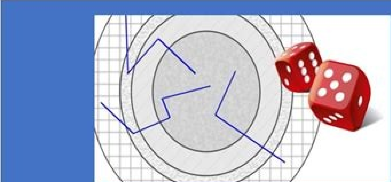
Ejemplo del método de Montecarlo en hoja de cálculo (Tutorial)
